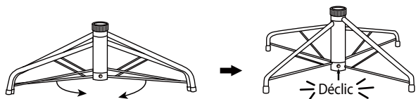
Fig. A – Assemblage du support d'arbre
