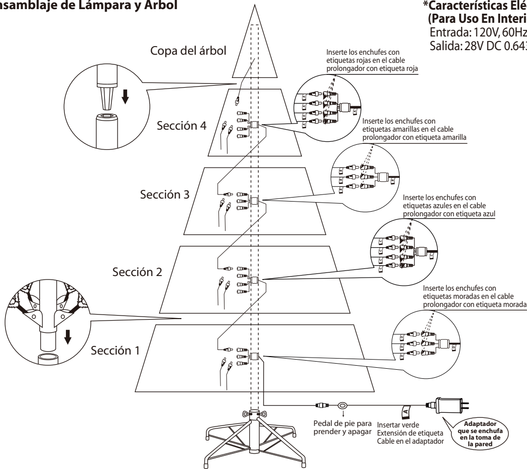
Fig. B - Ensamblaje de Lámpara y Árbol
