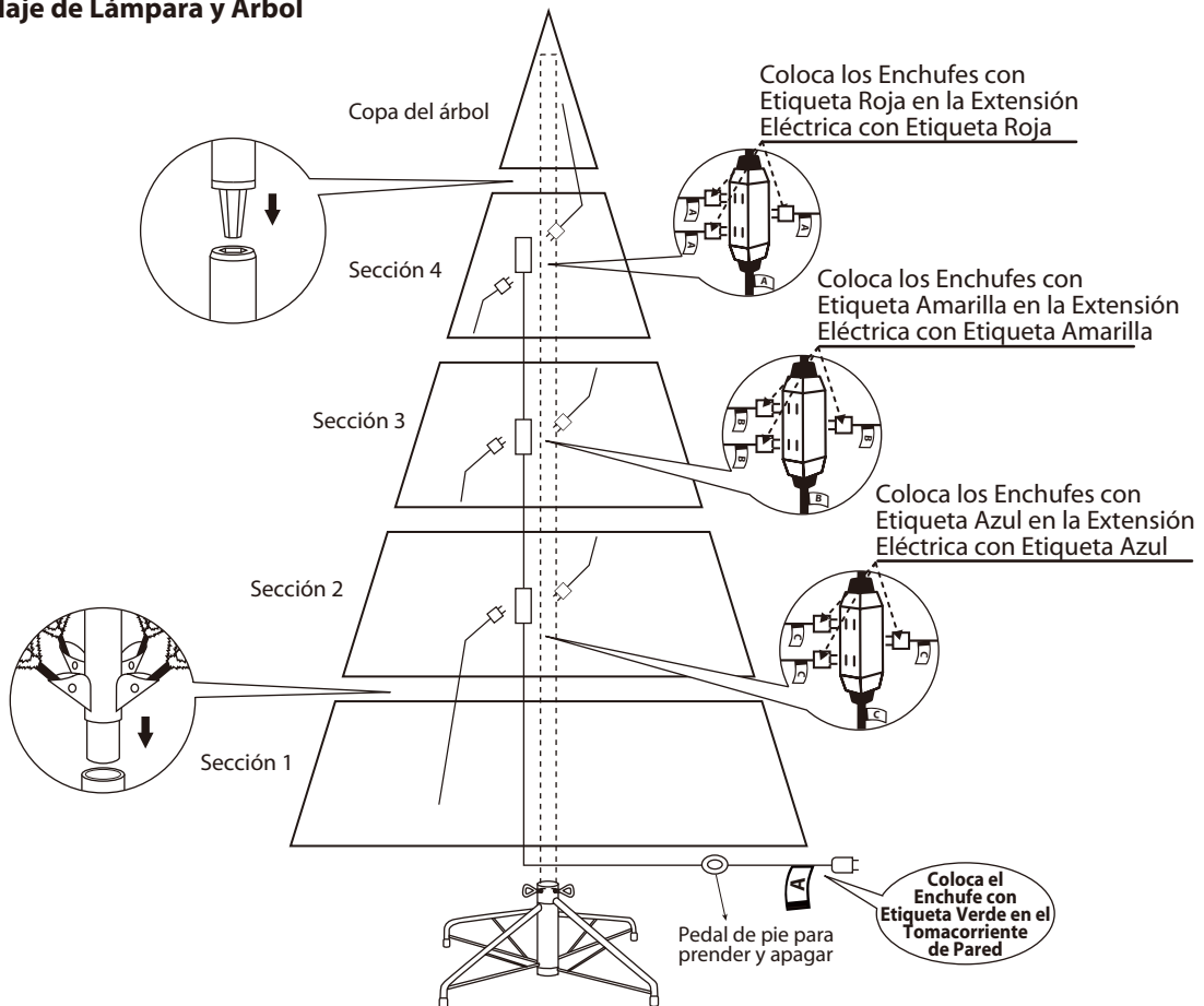
Fig. B - Ensamblaje de Lámpara y Árbol
