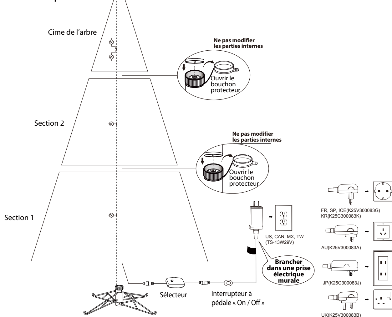
Figure B – Assemblage de l'arbre et des ampoules
